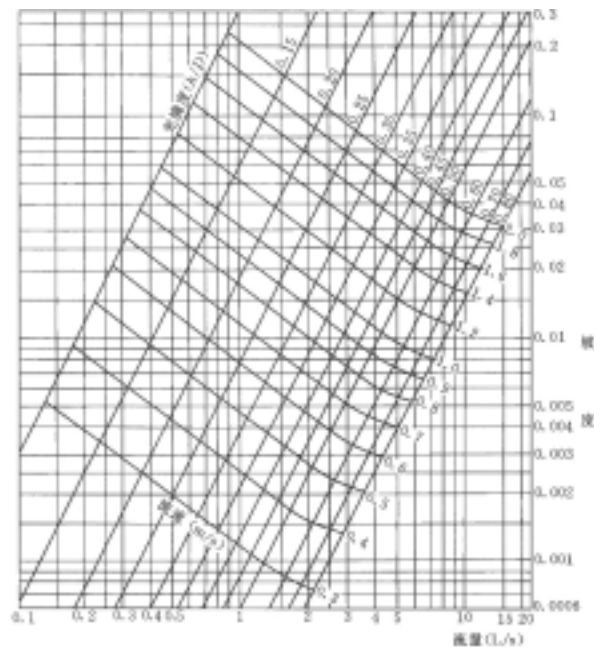
附图 A. 0.4 管径 110mm×3.2mm 横管计算图
