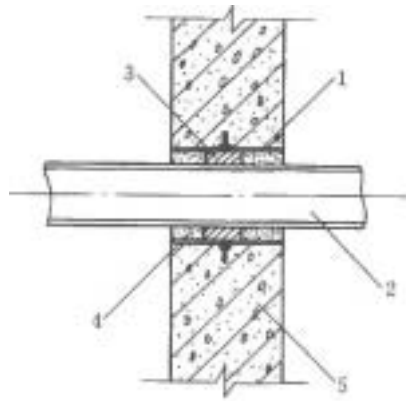
图 4.4.6 管道穿越地下室外墙
