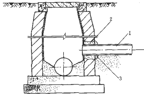
图 4.4.7 埋地管与检查井接点
