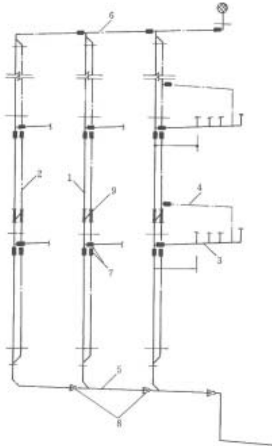
图 3.1.19 排水管、通气管设置伸缩节位置
