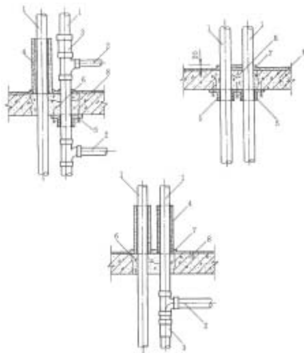
图 4.1.14—1 立管穿越楼层阻火圈、防火套管安装
