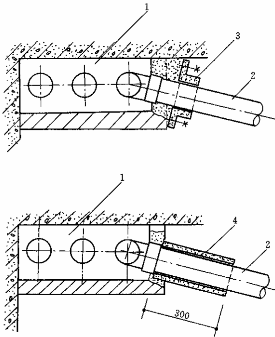
图 4.1.14-2 横支管接入管道井中立管阻火圈、 防火套管安装 1—管道井；2—PVC-U 横支管；3—阻火圈；4—防火套管
