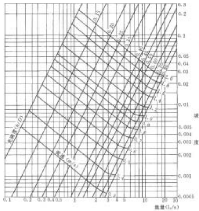
附图 A. 0.5 管径 125mm×3.2mm 横管计算图
