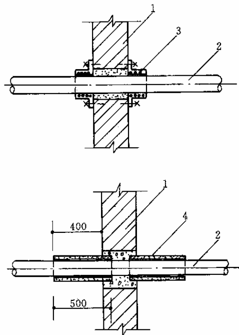
图 4.1.14-3 管道穿越防火分区隔墙阻火圈、 防火套管安装 1—墙体；2—PVC-U 横管；3—阻火圈；4—防火套管
