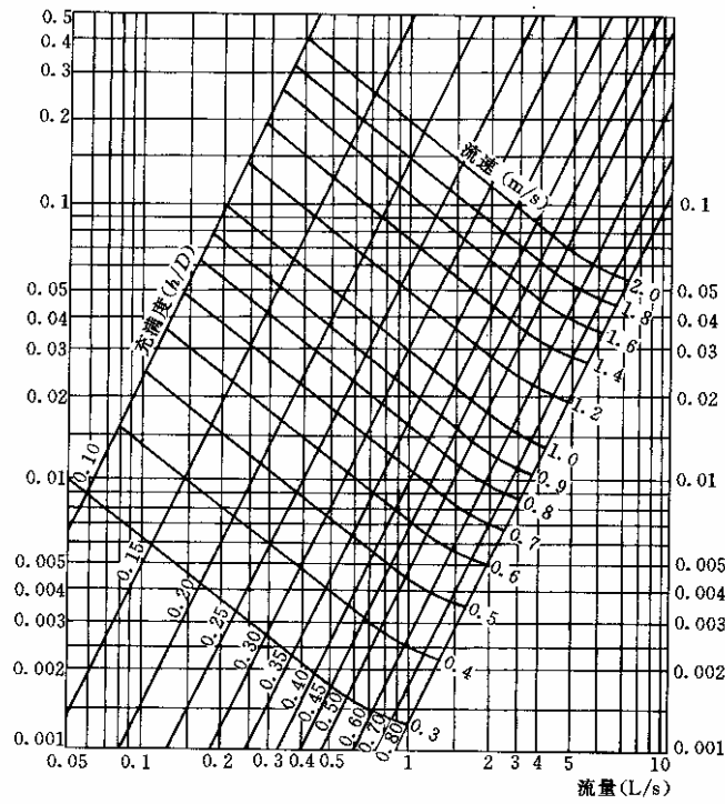
附图 A.0.2 管径 75mm×2.3mm 横管计算图
