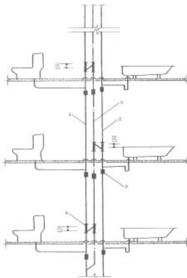
图1 H管件设置示意图
