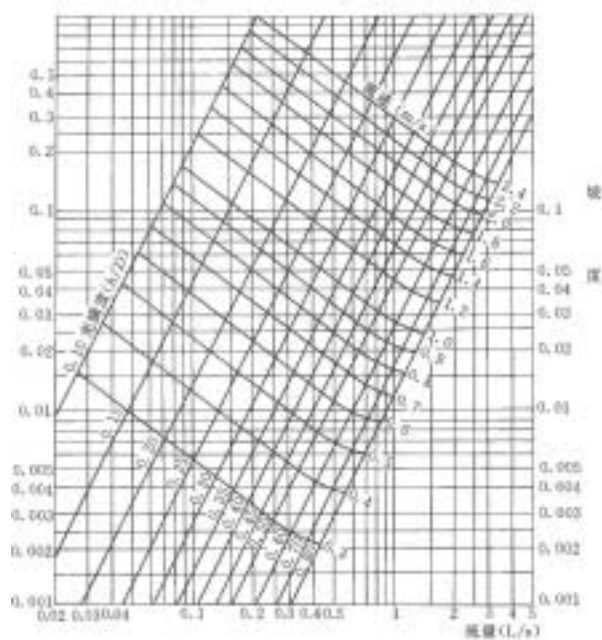
附图 A-0.1 管径 50mm×2mm 横管计算图
