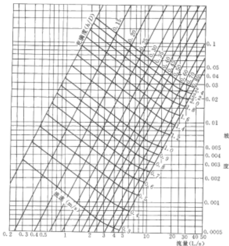
附图 A.0.6 管径 160mm×4mm 横管计算图
