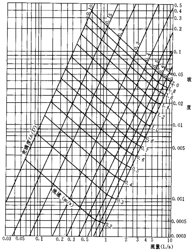
附图 A.0.3 管径 90mm×3.2mm 横管计算图
