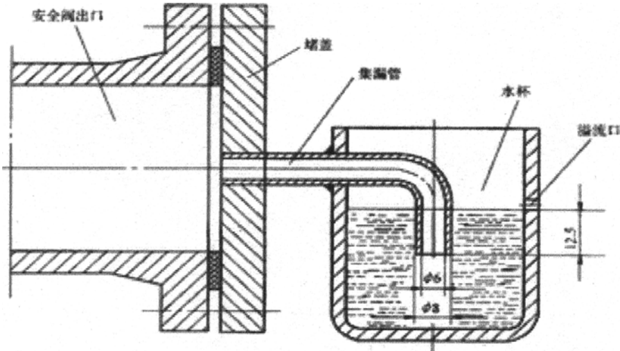
图 F—I 检漏方法示意
